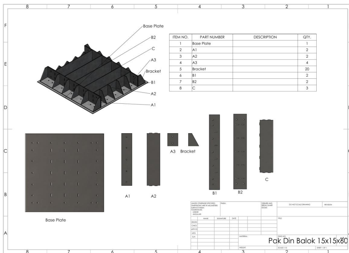
Gambar 1. Gambar teknik dan komponen konfigurasi cetakan balok
