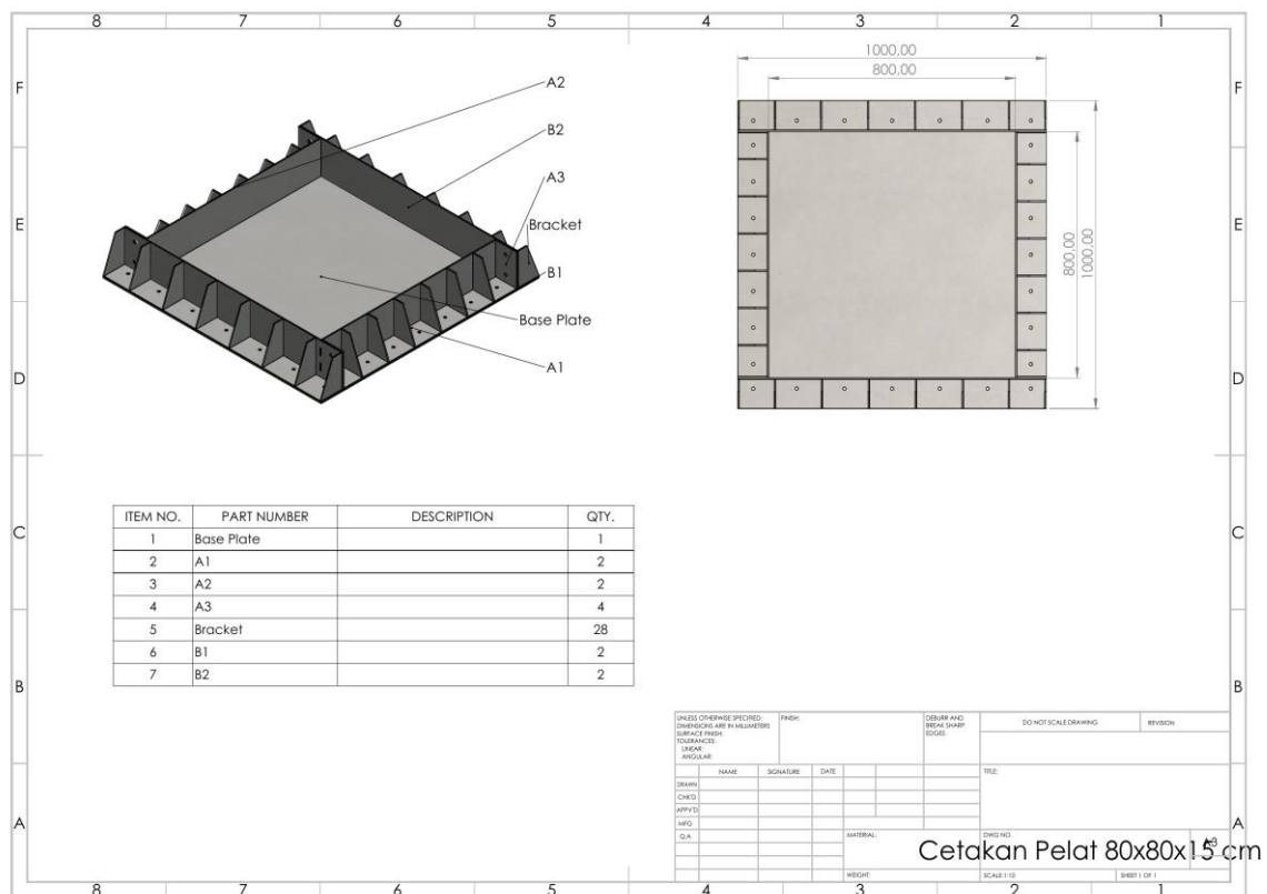
Gambar 2. Gambar teknik dan komponen konfigurasi cetakan pelat
